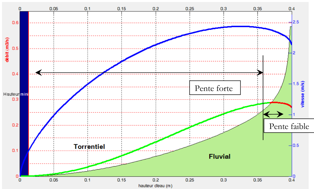
Figure 15. Domaines de fonctionnement hydraulique de la canalisation de décharge
