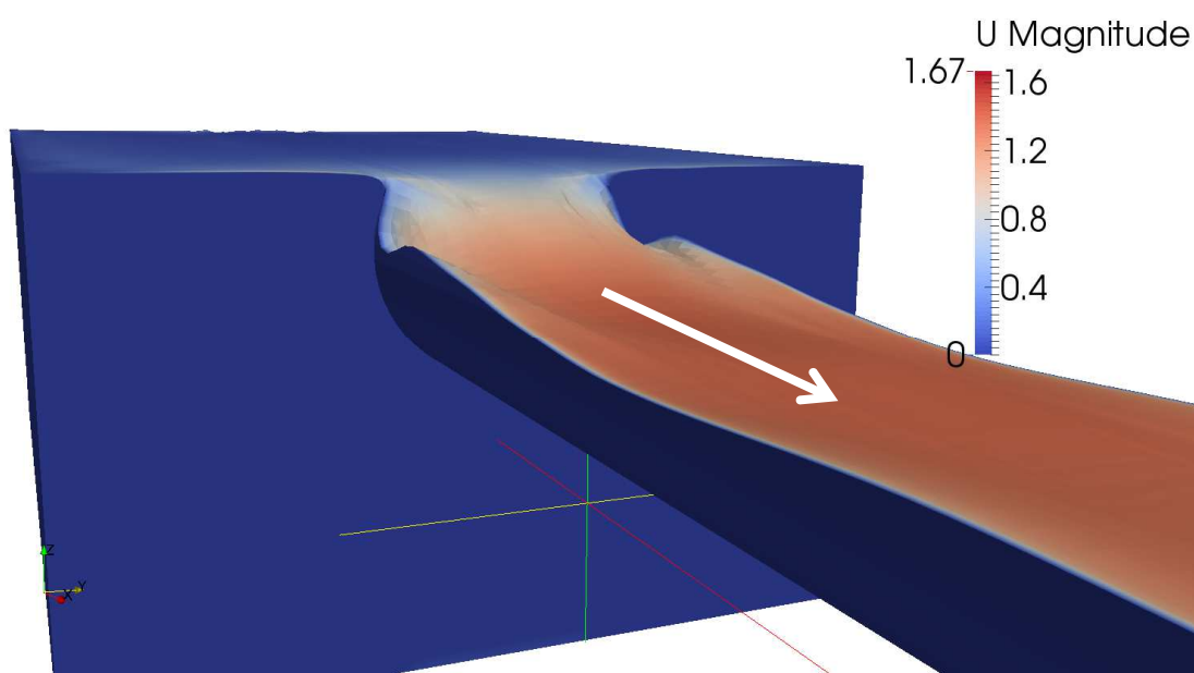
Figure 4. Vitesses au niveau de la surface libre - trop-plein en DN 300 et débit de 40 L/s
