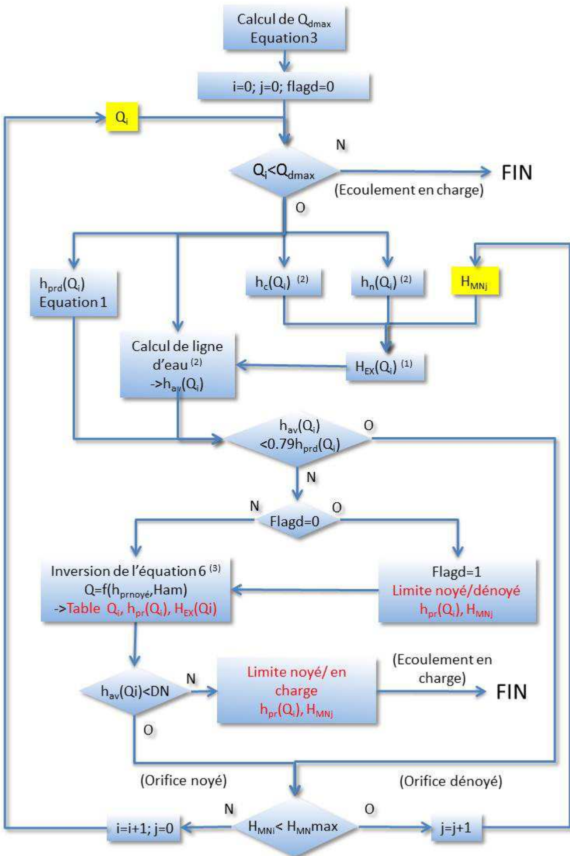
Figure 14. Logigramme général de détermination des lois de débit et de leur domaine d'application
