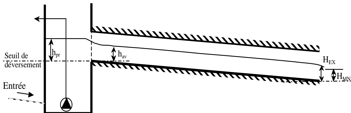
Figure 12. Variables et notations utilisées pour le couplage orifice-canalisation de décharge
