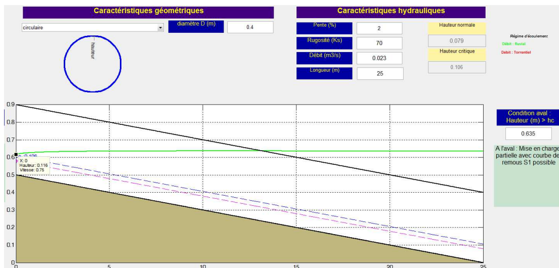
Figure 17. Calcul de ligne d'eau par le logiciel HSL
