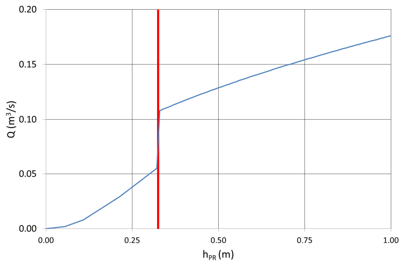
Figure 24. Débit surversé en fonction de h_{pr}
