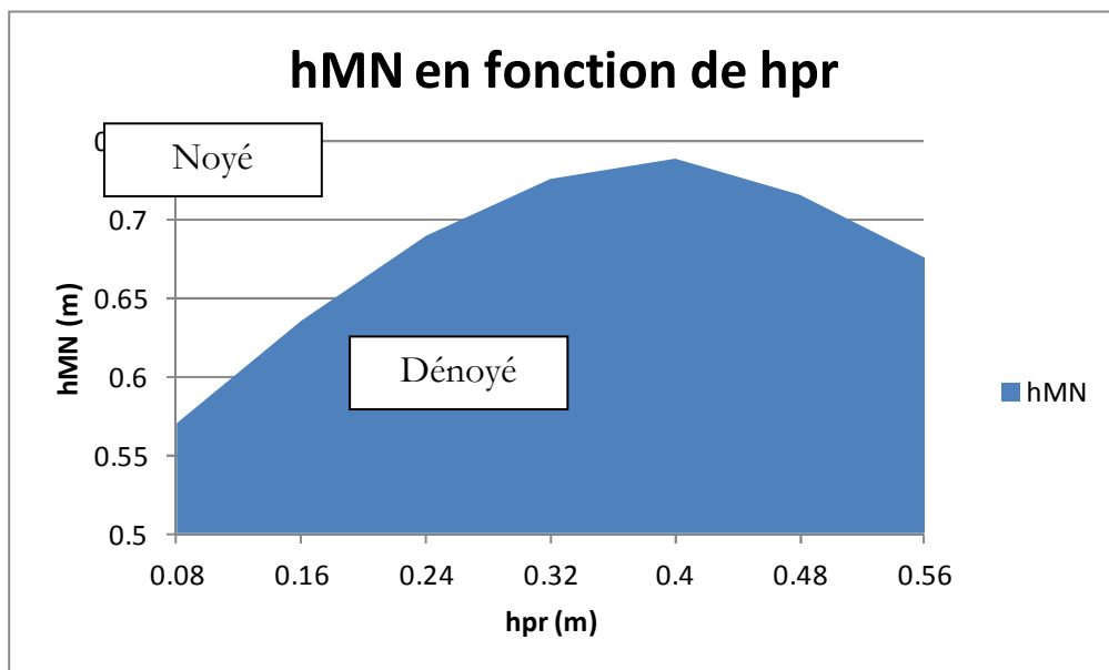
Figure 18. Domaines de fonctionnement en orifice noyé ou dénoyé
