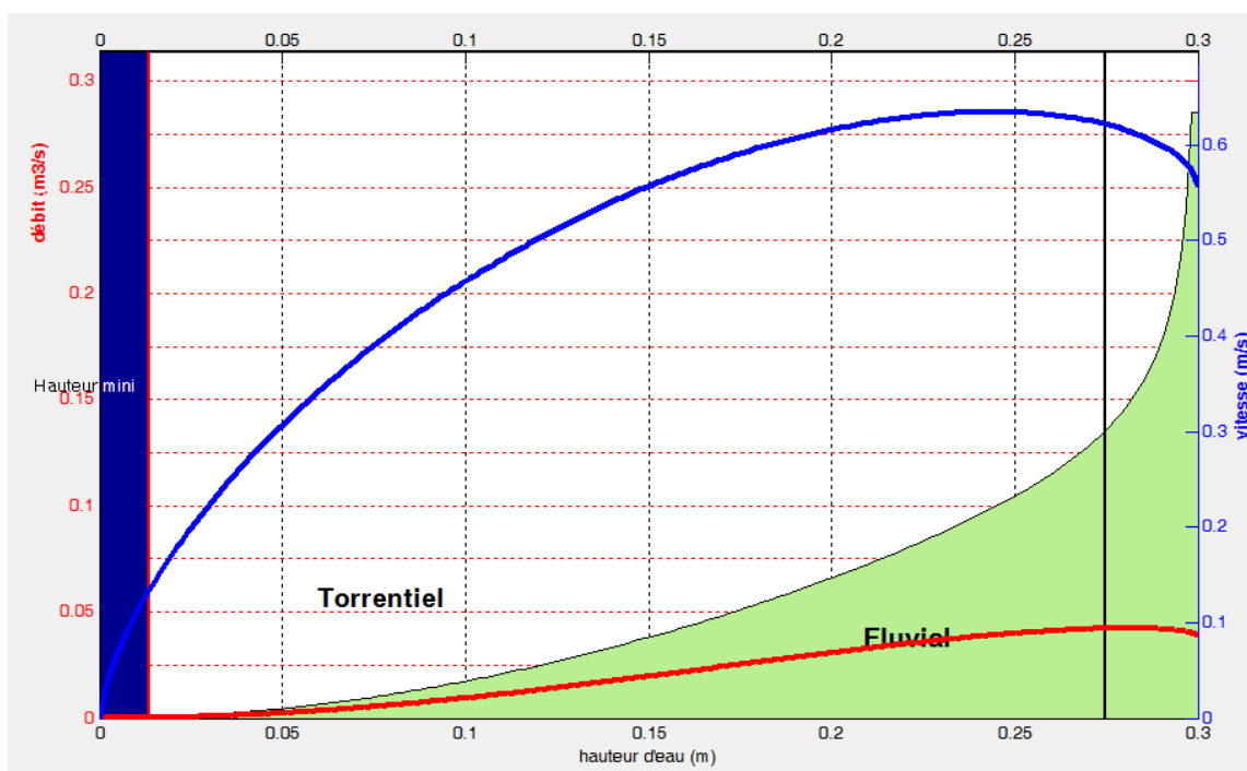
Figure 19. Domaines de fonctionnement hydraulique de la canalisation de décharge
