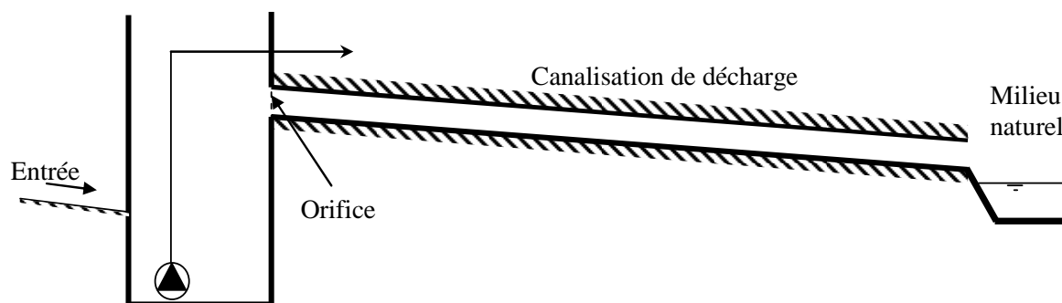
Figure 2. Profil en long d'un trop-plein de station de pompage
