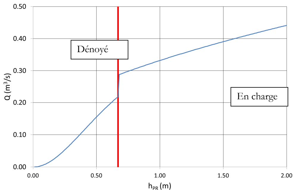
Figure 16. Débit surversé en fonction de h_{pr}
