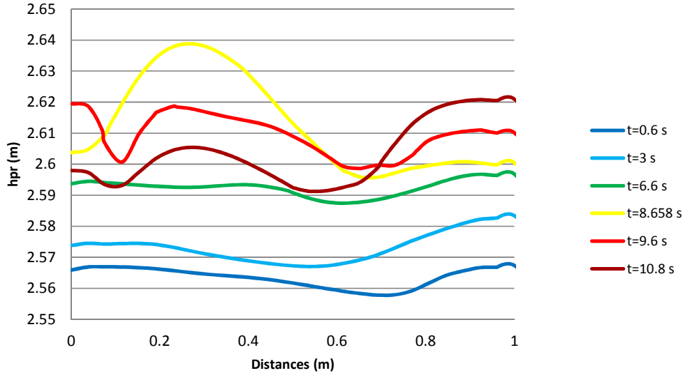
Figure 27. Variation de la hauteur d'eau dans la chambre au cours du temps.
