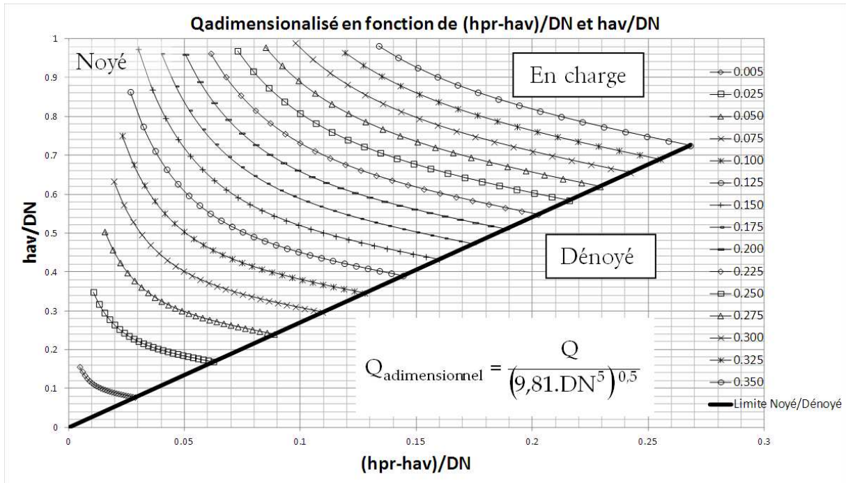
Figure 11. Abaque donnant le débit adimensionnel en fonction de la hauteur d'eau au-dessus du seuil de déversement et de la hauteur d'eau à l'aval immédiat de l'orifice Cas 3
