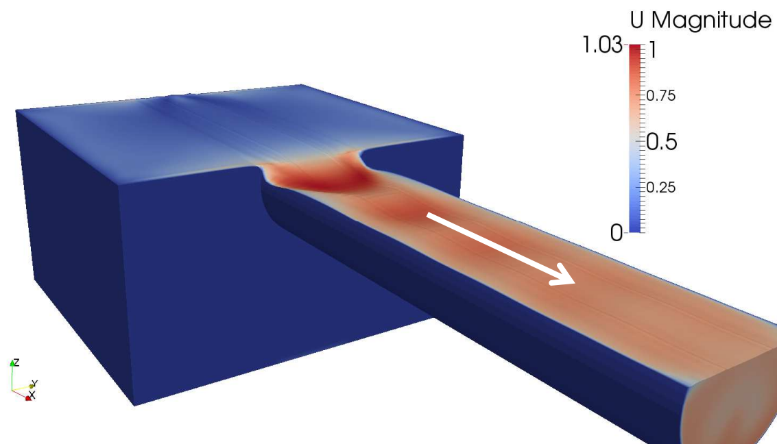
Figure 6. Trop-plein en DN 500 et débit de 86 L/s avec influence aval
