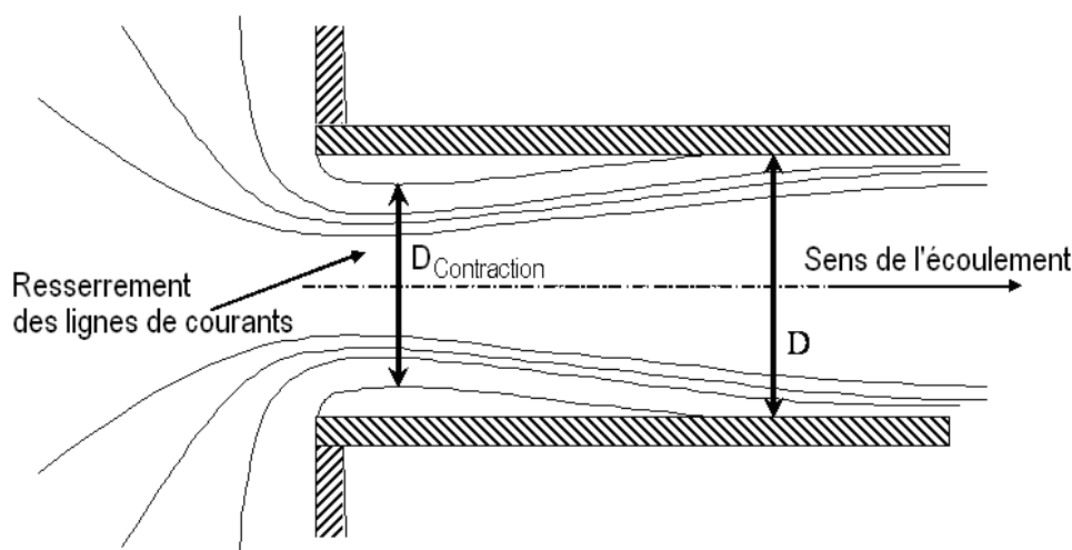
Figure 7. Contraction de la veine liquide au voisinage de la hauteur critique, vue de dessus
