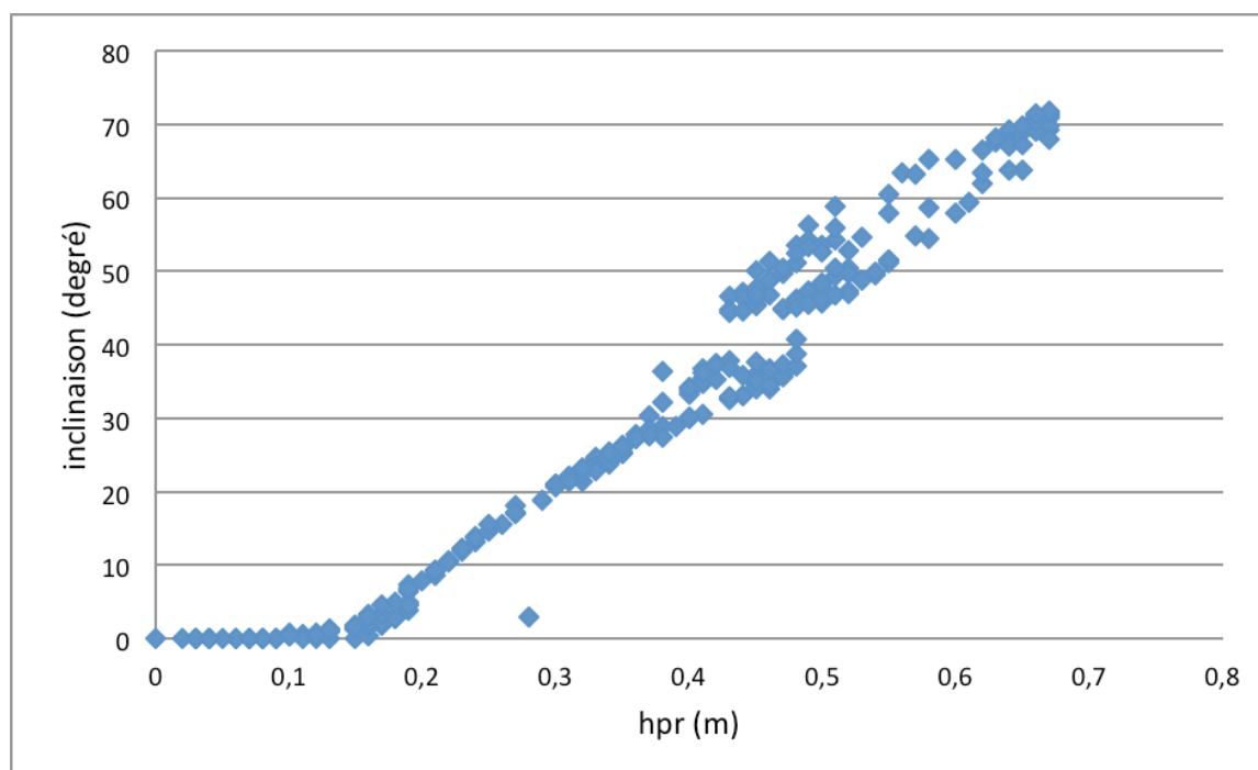
Figure 25. Relation entre l'inclinaison du clapet anti-retour et les hauteurs d'eau (données brutes) dans la chambre de relèvement (source : Jérôme de Bénédictis, Veolia Eau)
