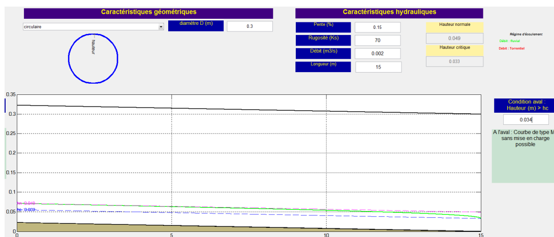
Figure 20. Ligne d'eau pour un débit de 2L/s
