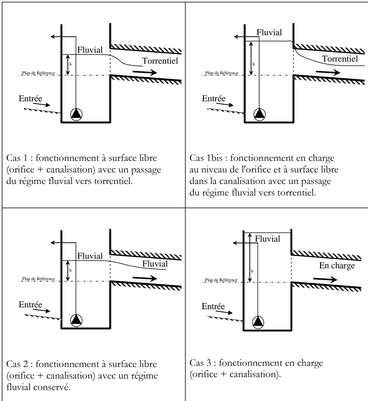
Figure 3. Modes de fonctionnement d'une surverse
