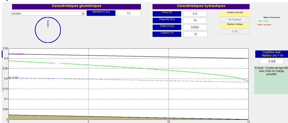
Figure 22. Ligne d'eau pour un débit de 55,3 L/s
