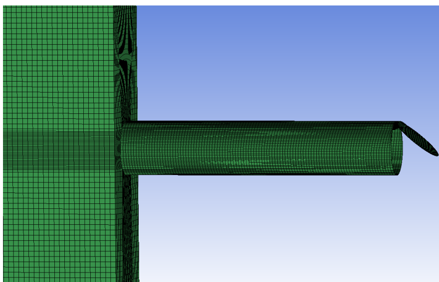
Figure 26. Géométrie et maillage du dispositif chambre-conduite-clapet (inclinaison de 50^\circ )
