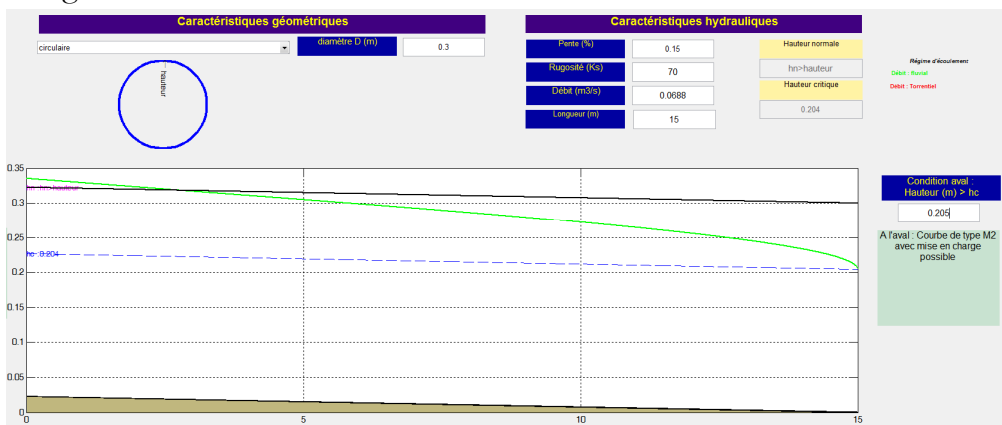
Figure 23. Ligne d'eau pour un débit de 68,8 L/s
