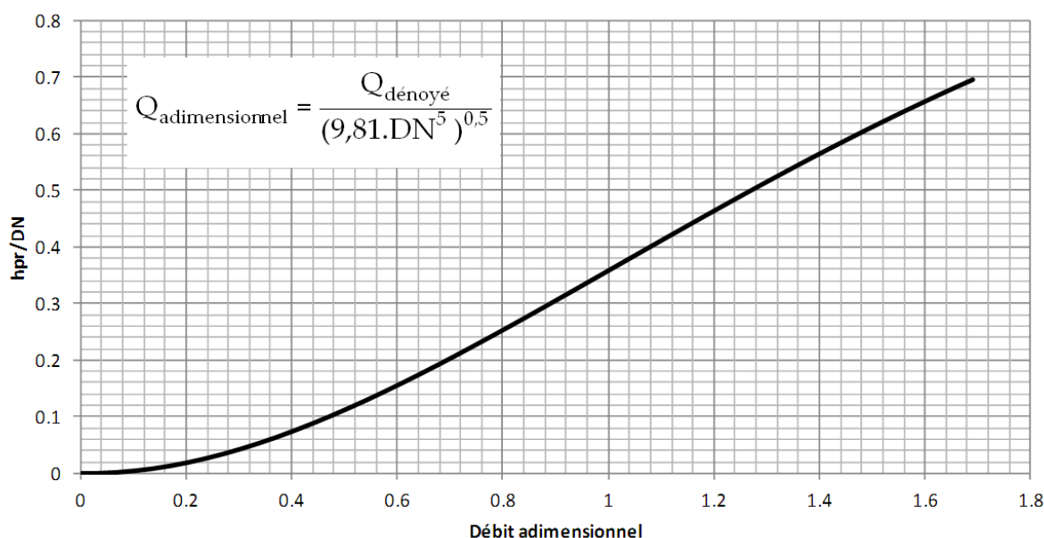
Figure 9. Evolution du débit adimensionnel en fonction de la hauteur d'eau au-dessus du seuil de déversement
