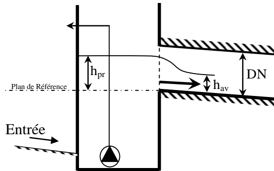
Figure 10. Représentation des variables de la formule de calcul pour le cas 2
