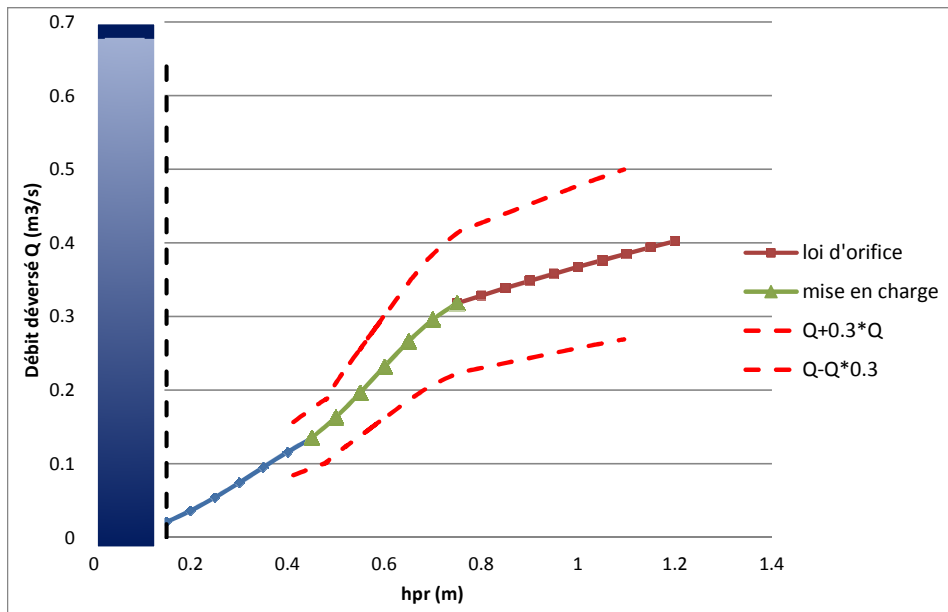
Figure 28. Courbes en pointillé rouge : évolution du débit en fonction de la hauteur d'eau dans la chambre pour le cas d'une conduite de surverse équipée d'un clapet ; Ligne verticale en noir : hauteur d'eau provoquant l'ouverture du clapet ; les autres courbes : évolution du débit en fonction de la hauteur d'eau dans la chambre en régime permanent sans prise en compte de la présence du clapet.
