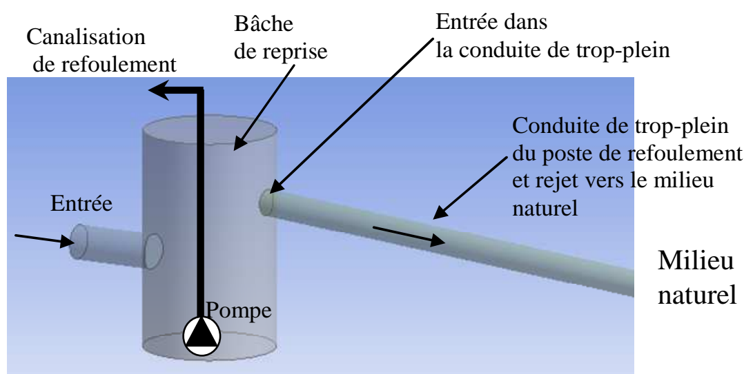
Figure 1. Composantes d'un trop-plein de station de pompage
