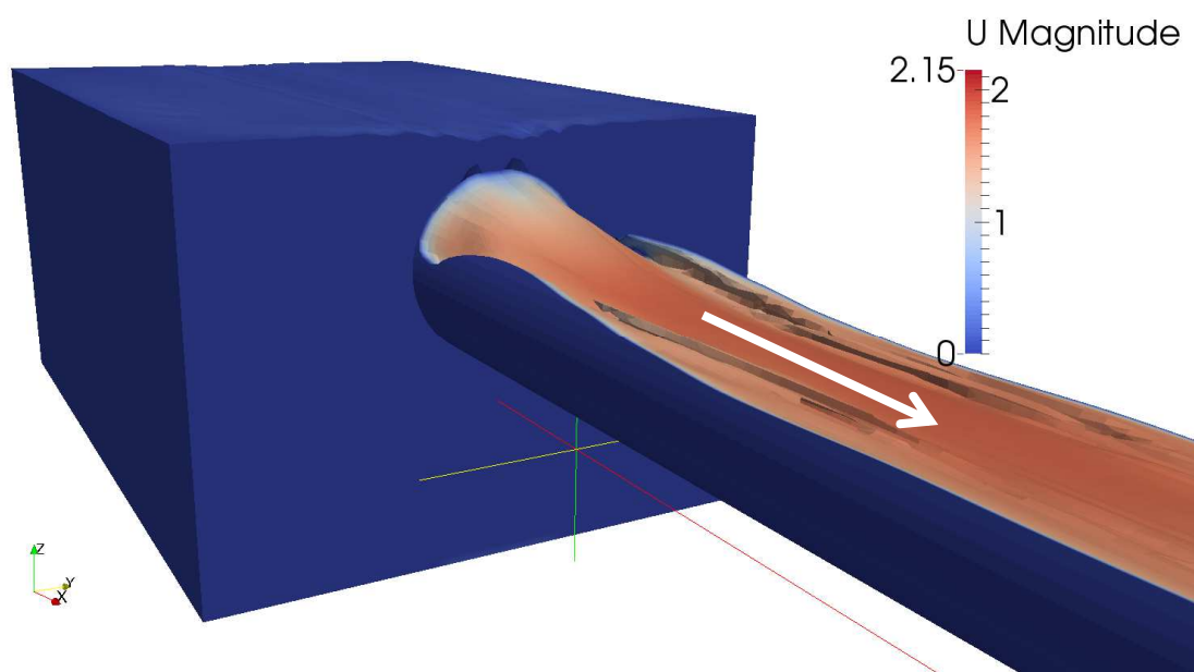
Figure 5. Trop-plein en DN 300 et débit de 75 L/s
