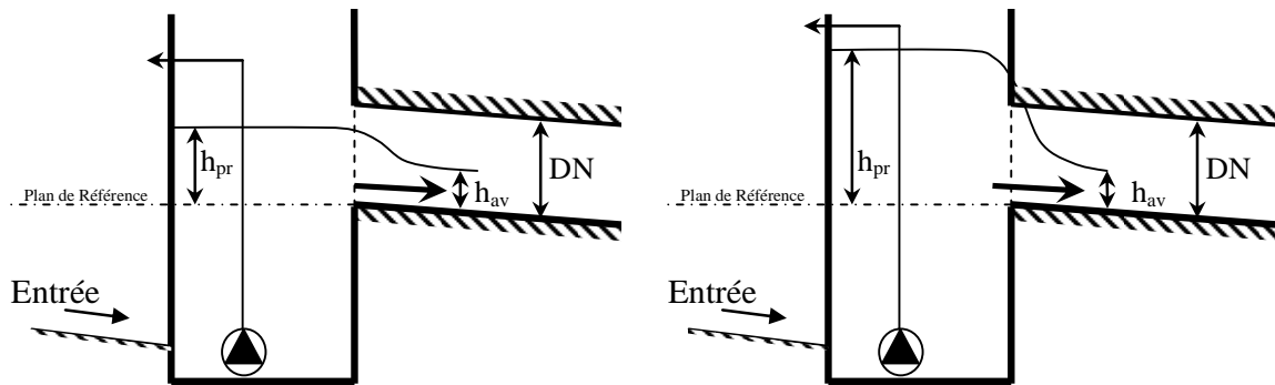
Figure 8. Représentation des variables de la formule de calcul pour les cas 1 et 1bis
